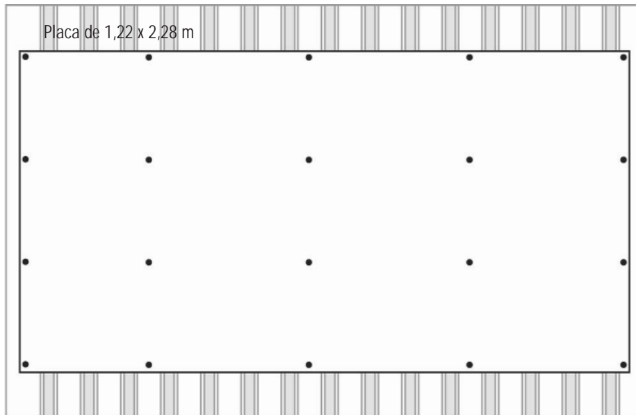
Figura B disposição dos parafusos da parte superior
